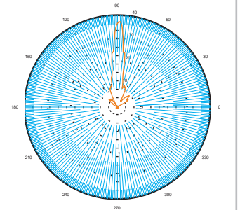
11.7 Ghz H-Plane
