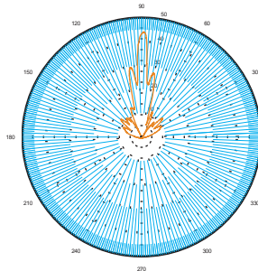
11.7 Ghz E-Plane
